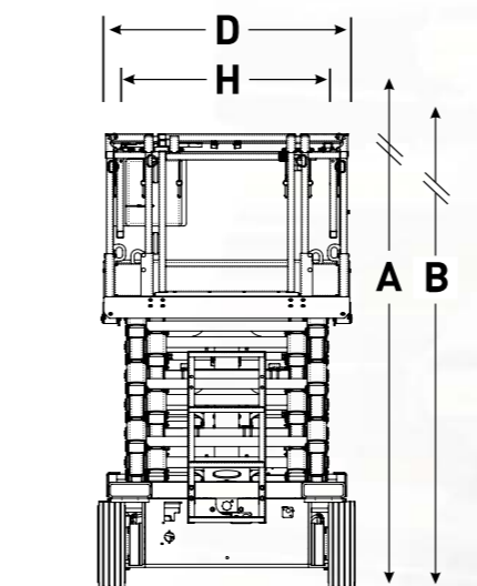
RÜCKANSICHT, EINGEFAHREN (GELÄNDER ZUSAMMENGEKLAFFT)
